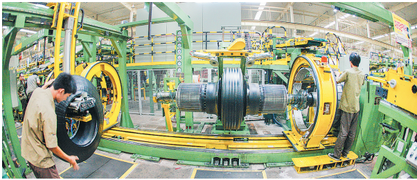
忙碌的风神轮胎工程胎生产线。
