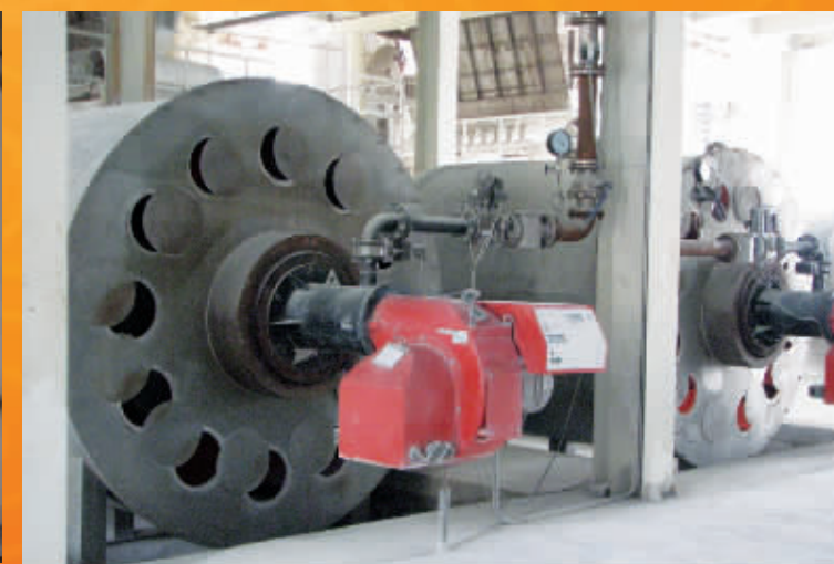
公司后处理车间一角
